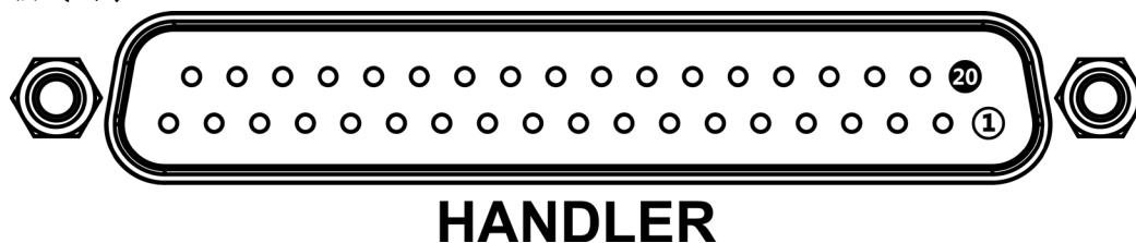
图 7-1 接线端子
