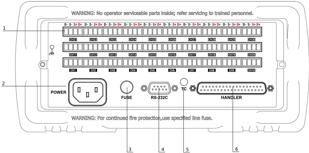
图 3-2 后面板
