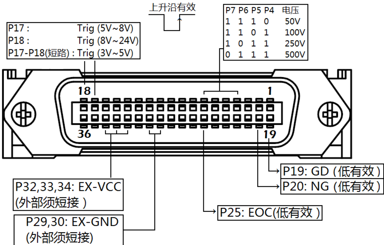
图 4-1 接线端子
