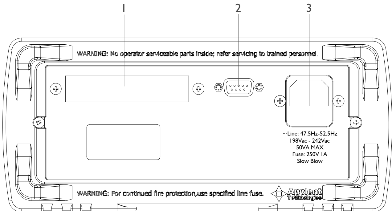
图 3-5 后面板
