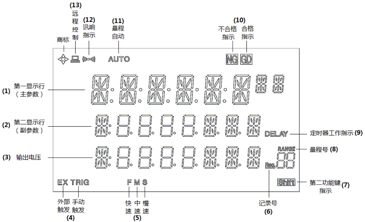
图 3-2 显示屏幕
