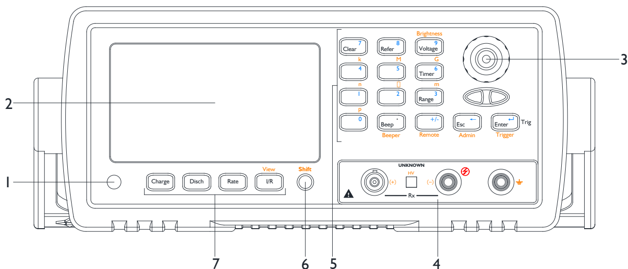
图 3-1 前面板
