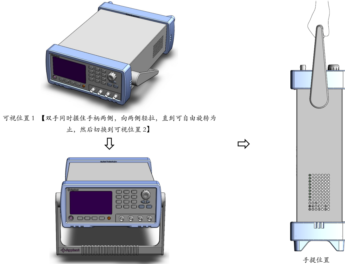
图 1-2 仪器手柄
