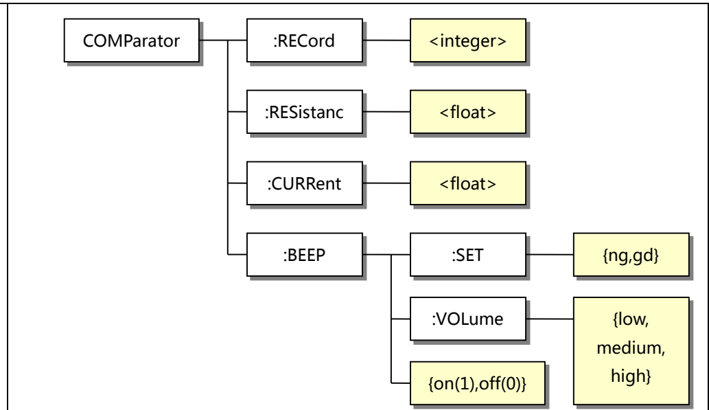
图 6-5 COMParator 命令树
