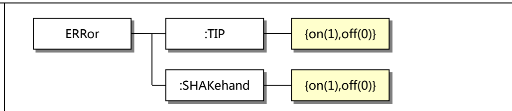
图 6-12 ERRor? 命令树
